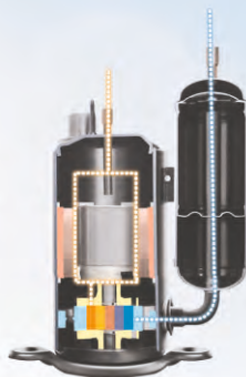
Обычный компрессор
