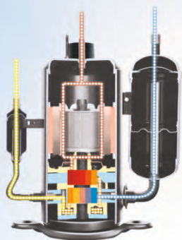
Двухступенчатый компрессор
